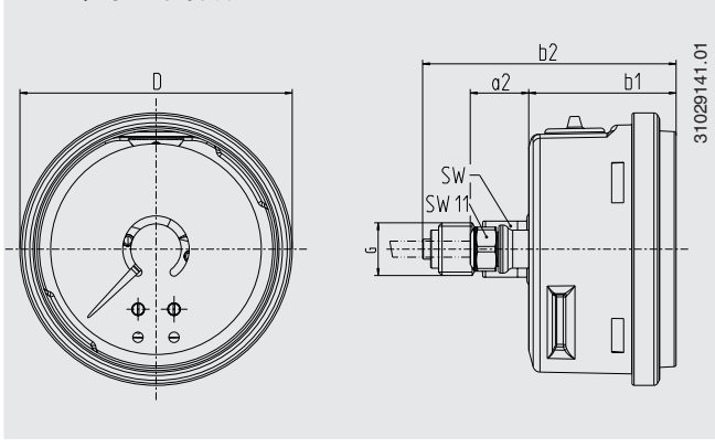
NS 50, 中心背部安装
